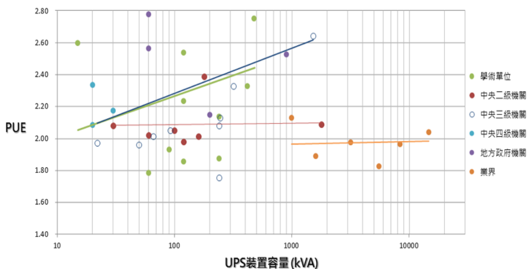
圖 1：政府機房能源使用效率量測結果
