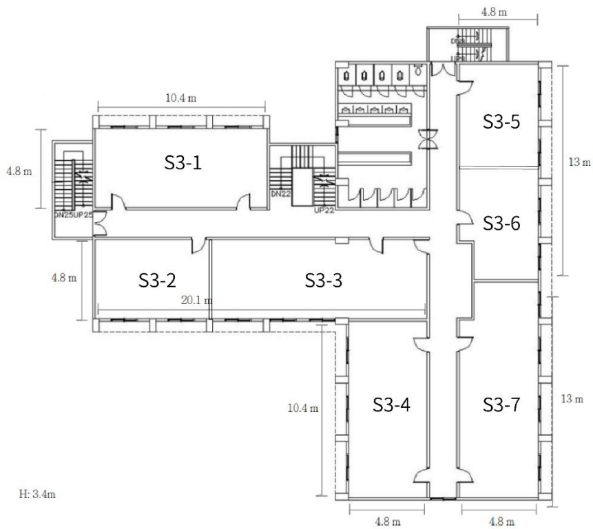
士官大樓 三樓平面圖
