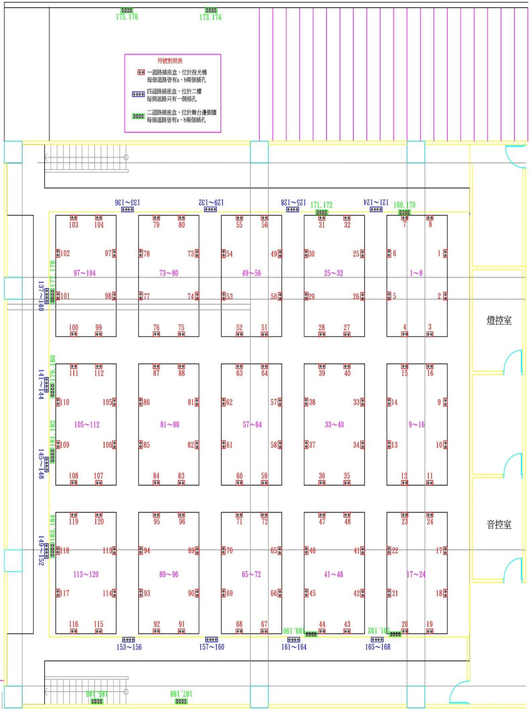
附圖 1 曲藝館燈光迴路號碼圖
