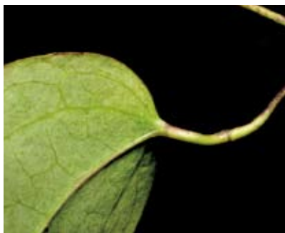
柱果鐵線蓮的小葉柄有關節
