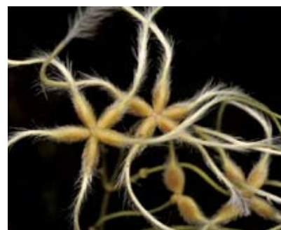
威靈仙的果實
