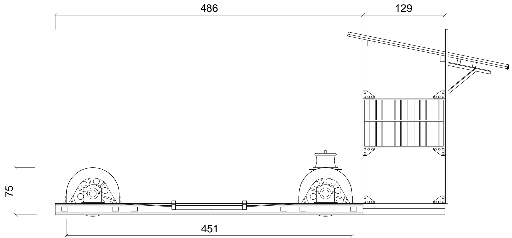
移車台西向立面圖
