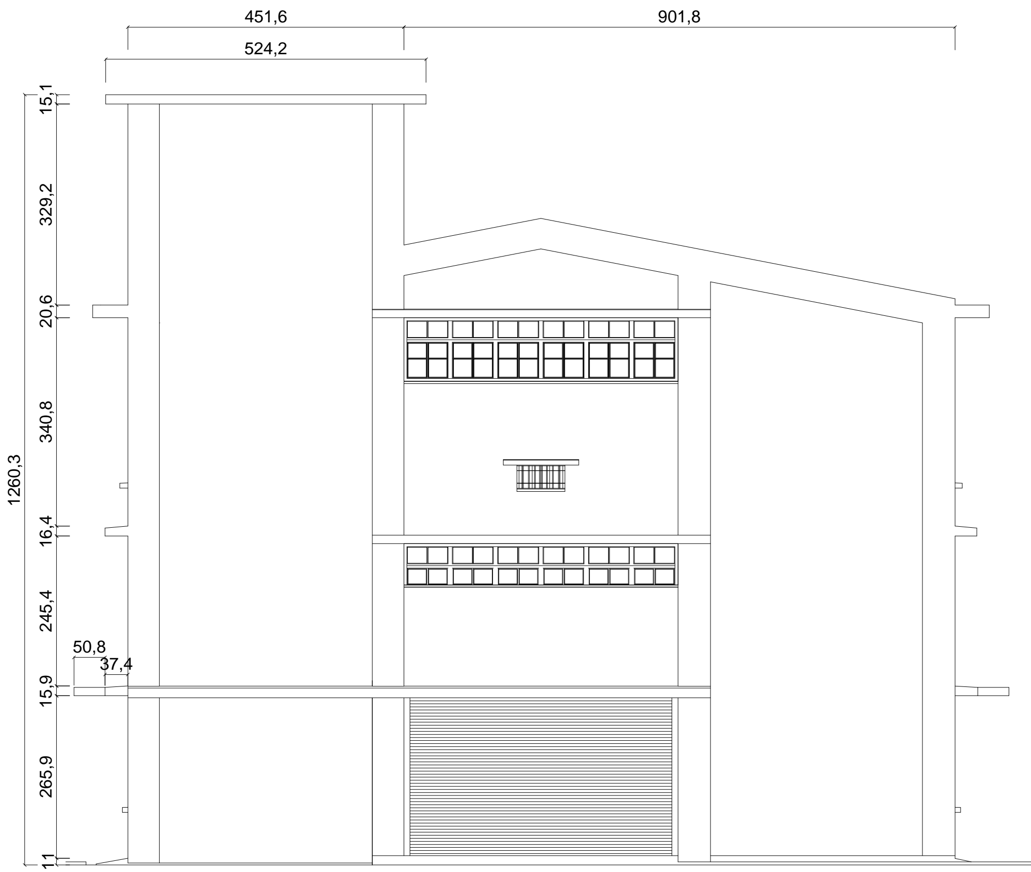
松山材料場(一)西向立面圖
