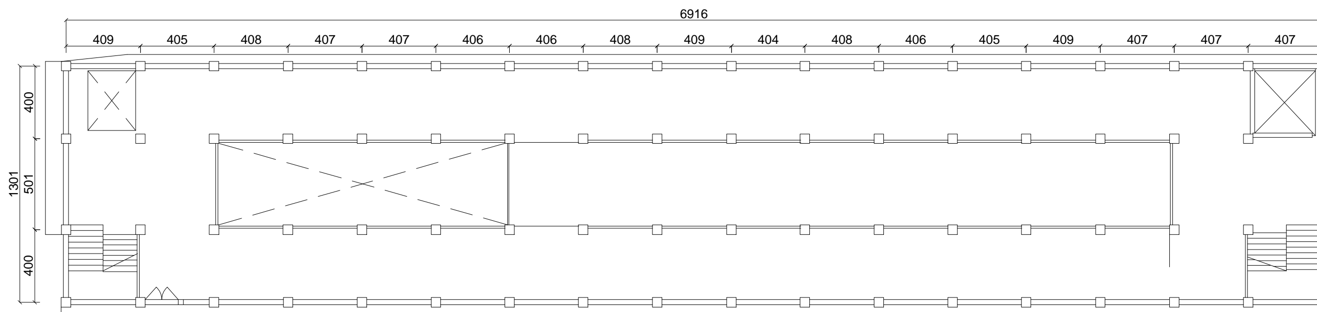
松山材料場(一)2F平面圖
