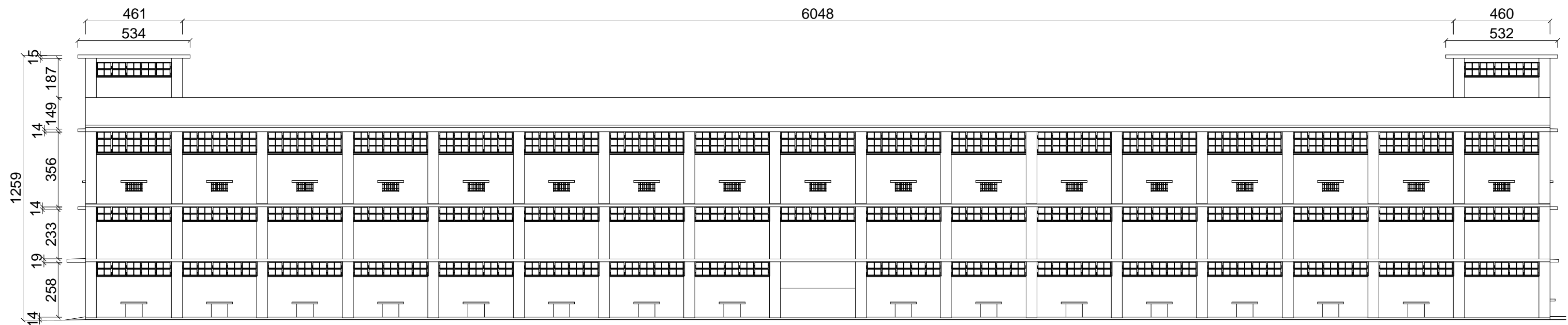
松山材料場(一)南向立面圖
