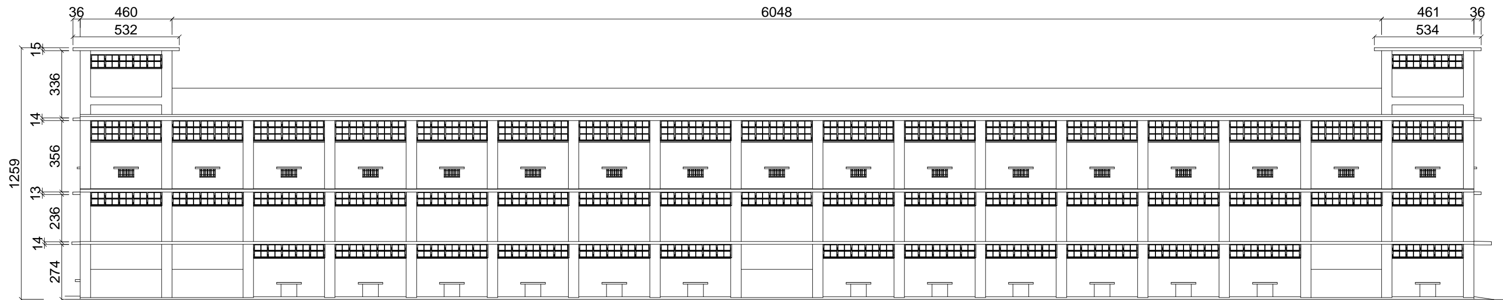
松山材料場(一)北向立面圖
