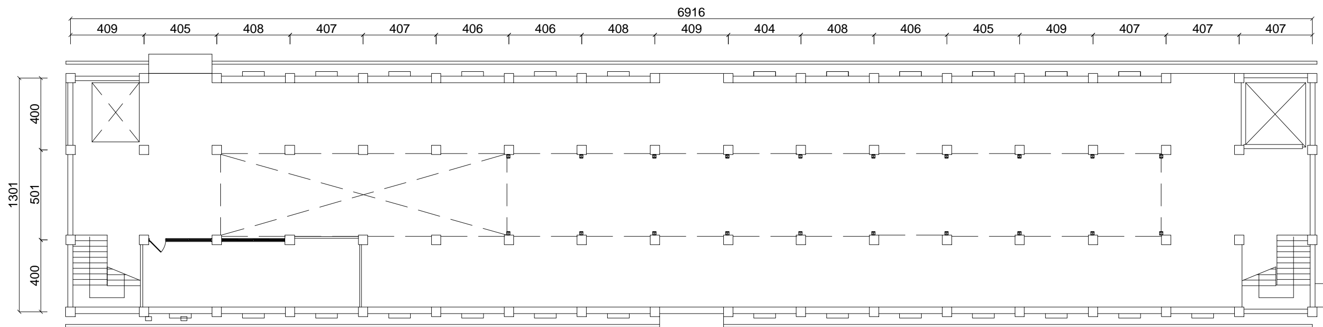
松山材料場(一)1F平面圖
