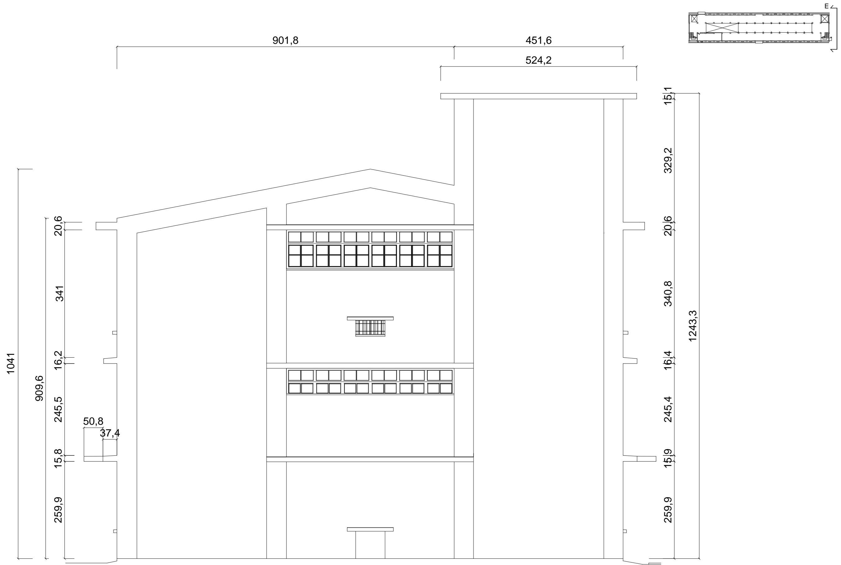
松山材料場(一)東向立面圖
