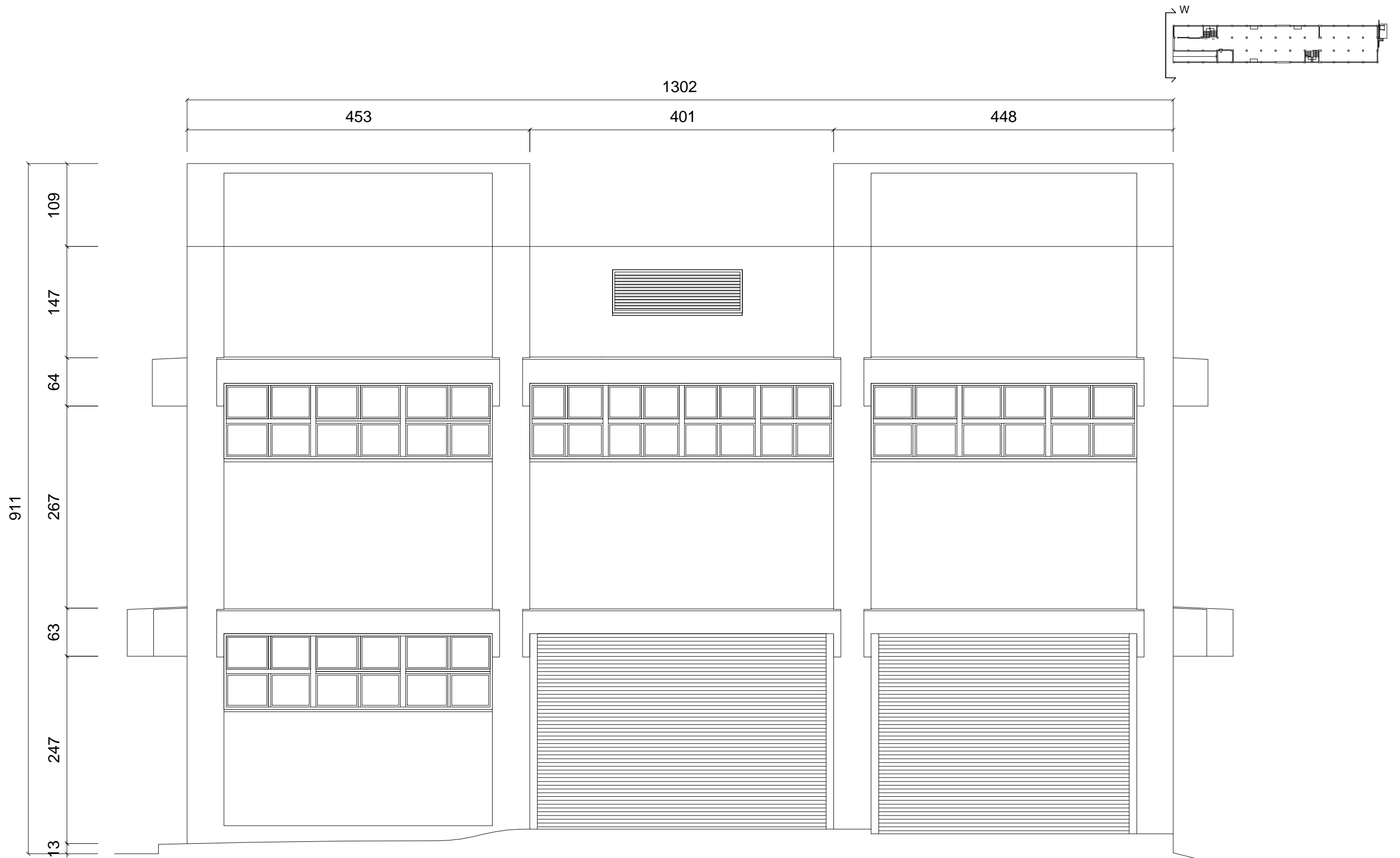
松山材料場(二)西向立面圖
