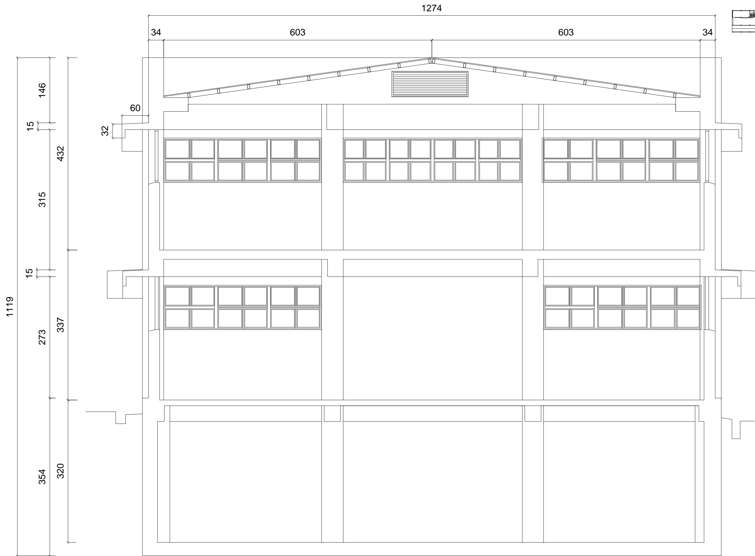
松山材料場(二)B-B'剖面圖
