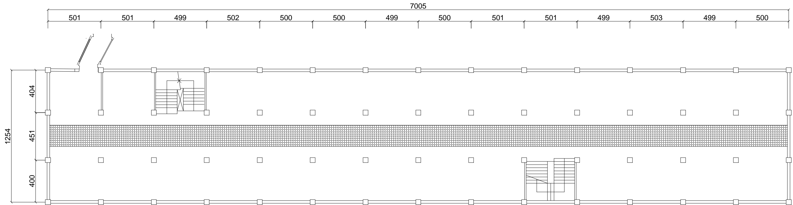
松山材料場(二)2F平面圖
