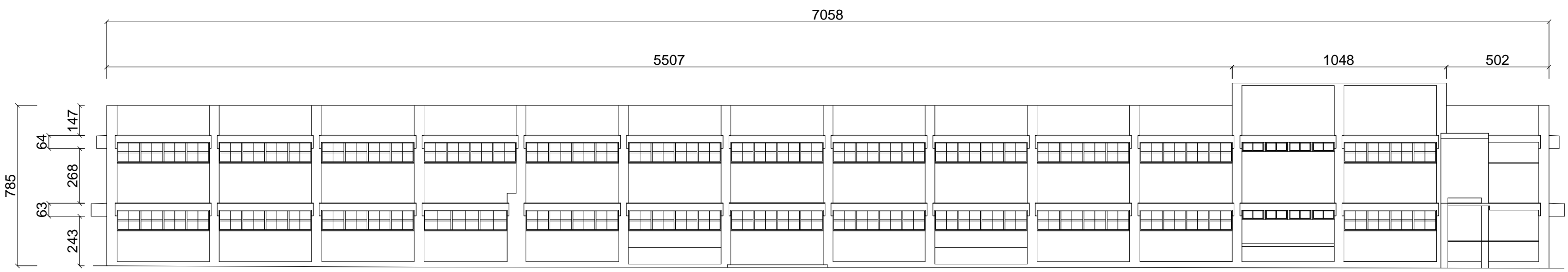
松山材料場(二)北向立面圖
