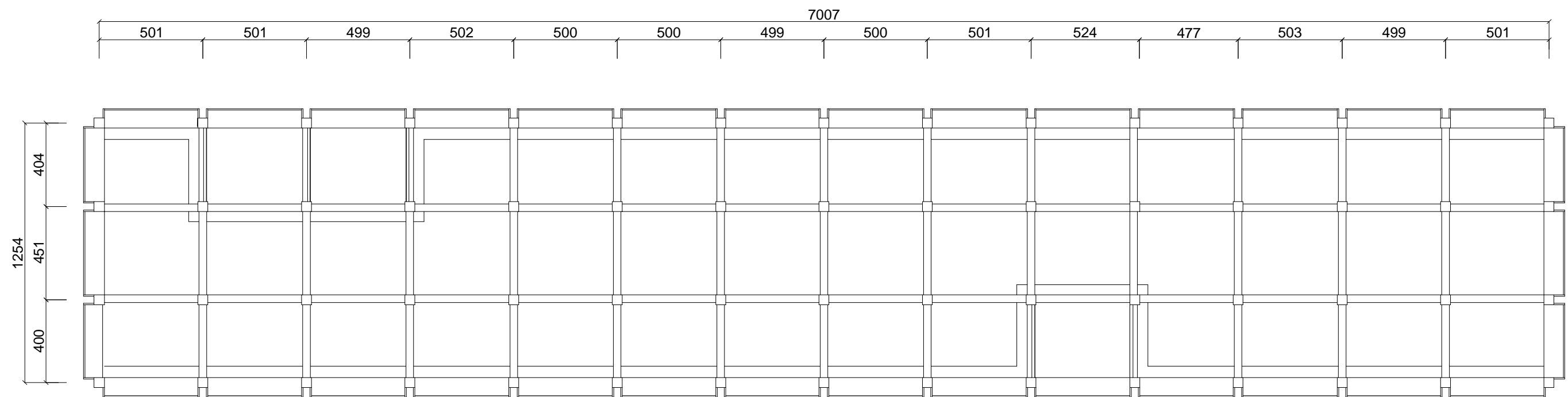
松山材料場(二)2F天花反射平面圖
