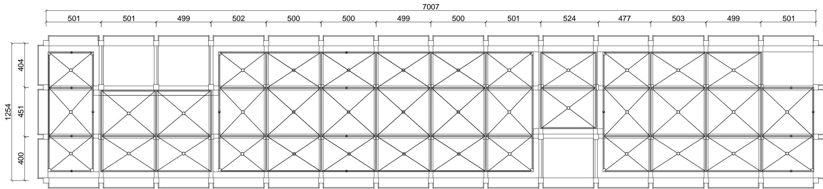
松山材料場(二)屋架反射平面圖(下層)
