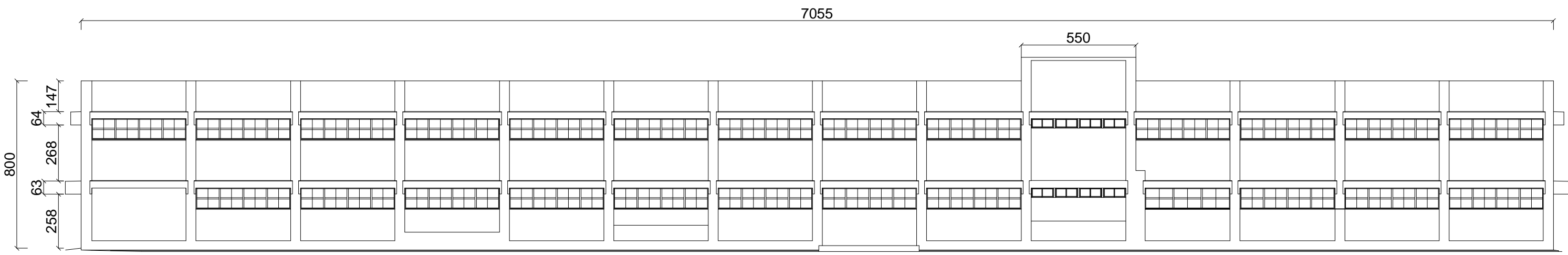
松山材料場(二)南向立面圖
