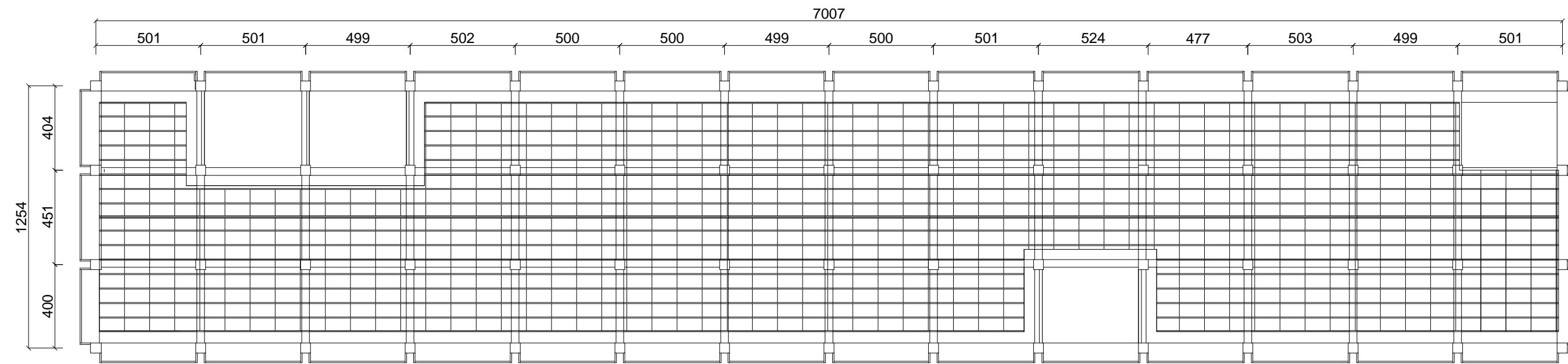
松山材料場(二)屋架反射平面圖(上層)
