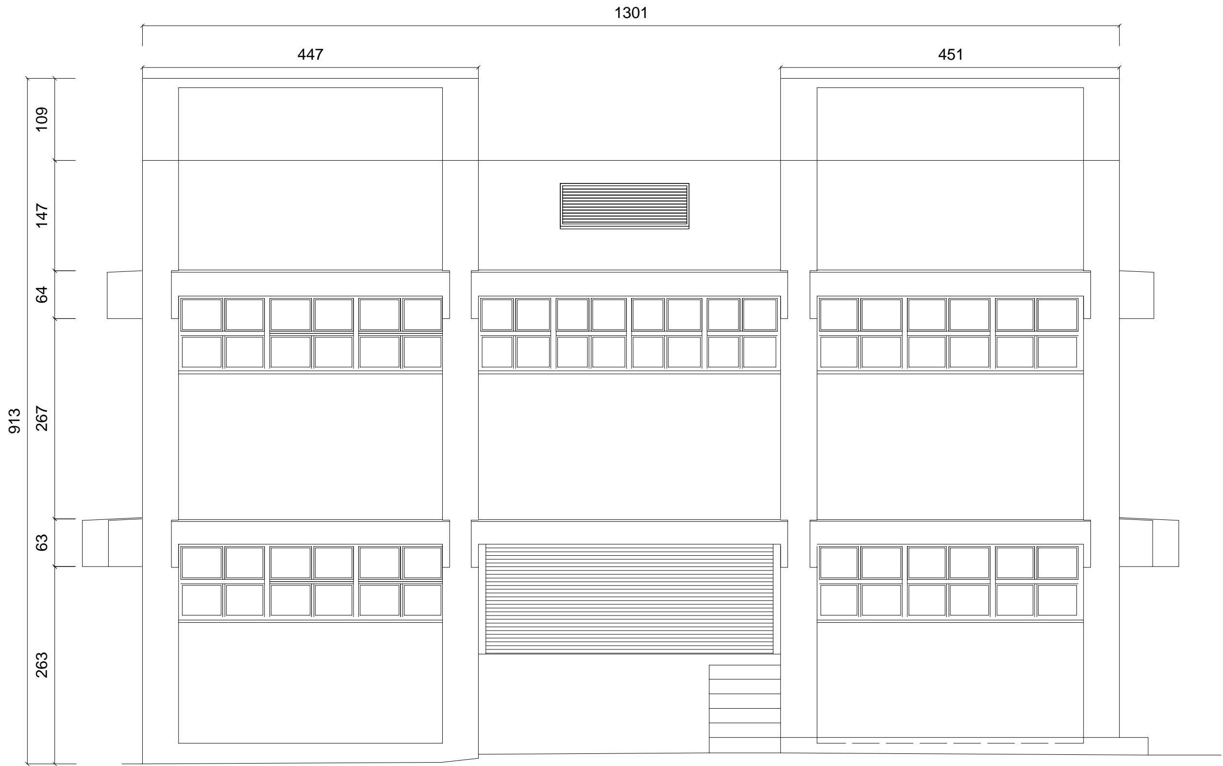
松山材料場(二)東向立面圖
